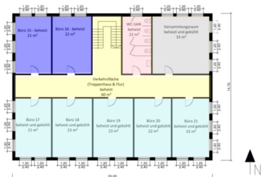
2.Obergeschoss
