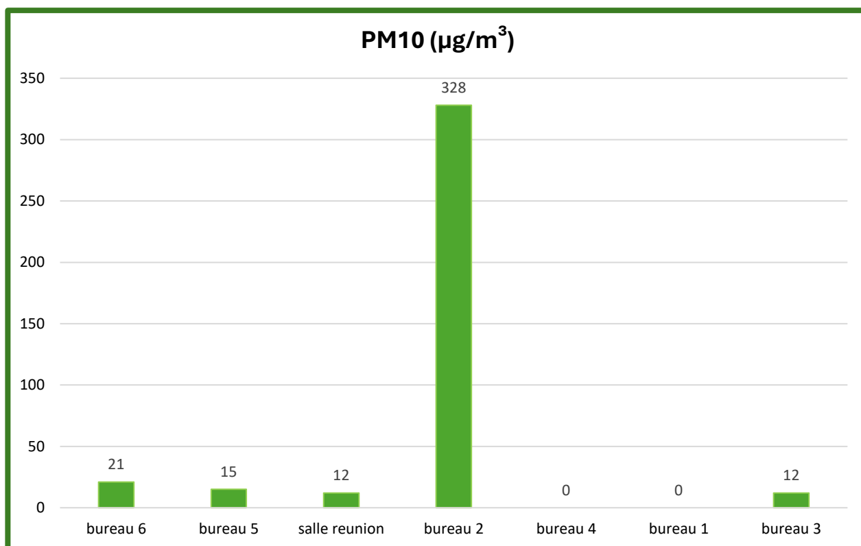
F 46 : Concentrations en PM10 : bâtiment fonctionnel à Copenhague 69
